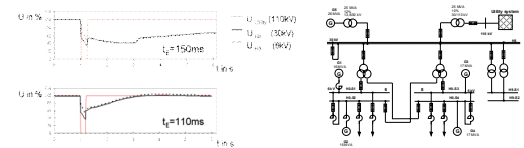
Abbildung 2: Spannungswiederkehr nach Kurzschluss in einem 110 kV Netz für 150 / 110 ms
