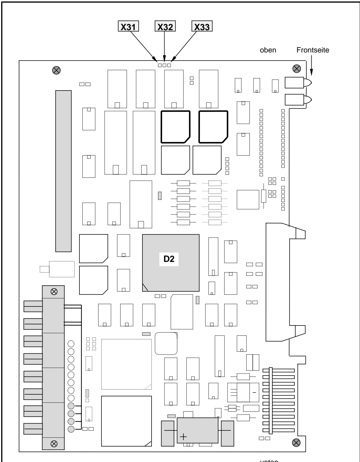
Bild 2: ZPH-Platine, Bestückungsseite Lage der Stifte X31, 32, X33 Lagedes ZPH-Prozessors D2
