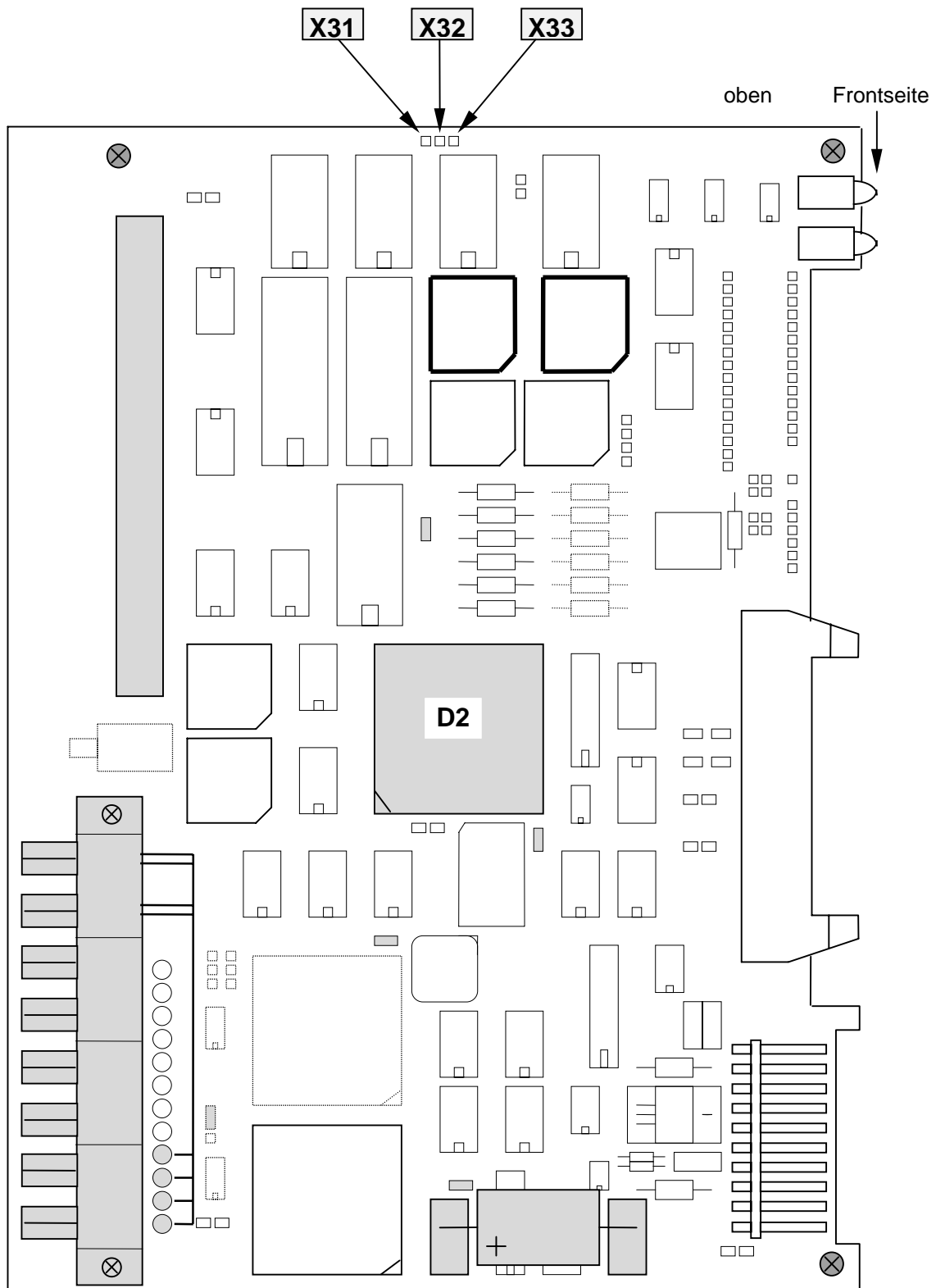
Bild 2: ZPH-Platine, Bestückungsseite Lage der Stifte X31, 32, X33 Lagedes ZPH-Prozessors D2
