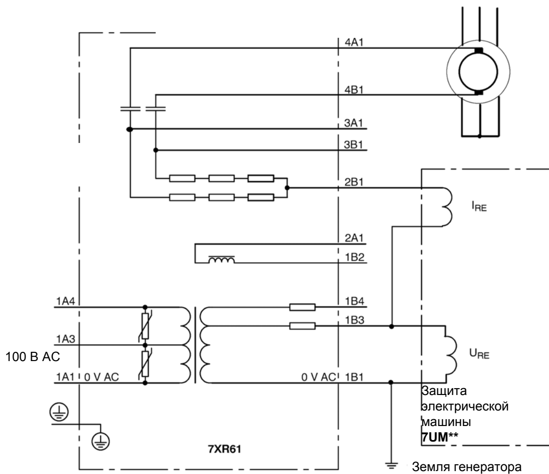
Рисунок 6 Пример подключения 1: среднеквадратичное значение тока на зажимах 4A1, 4B1 \leq 0,2 А AC
