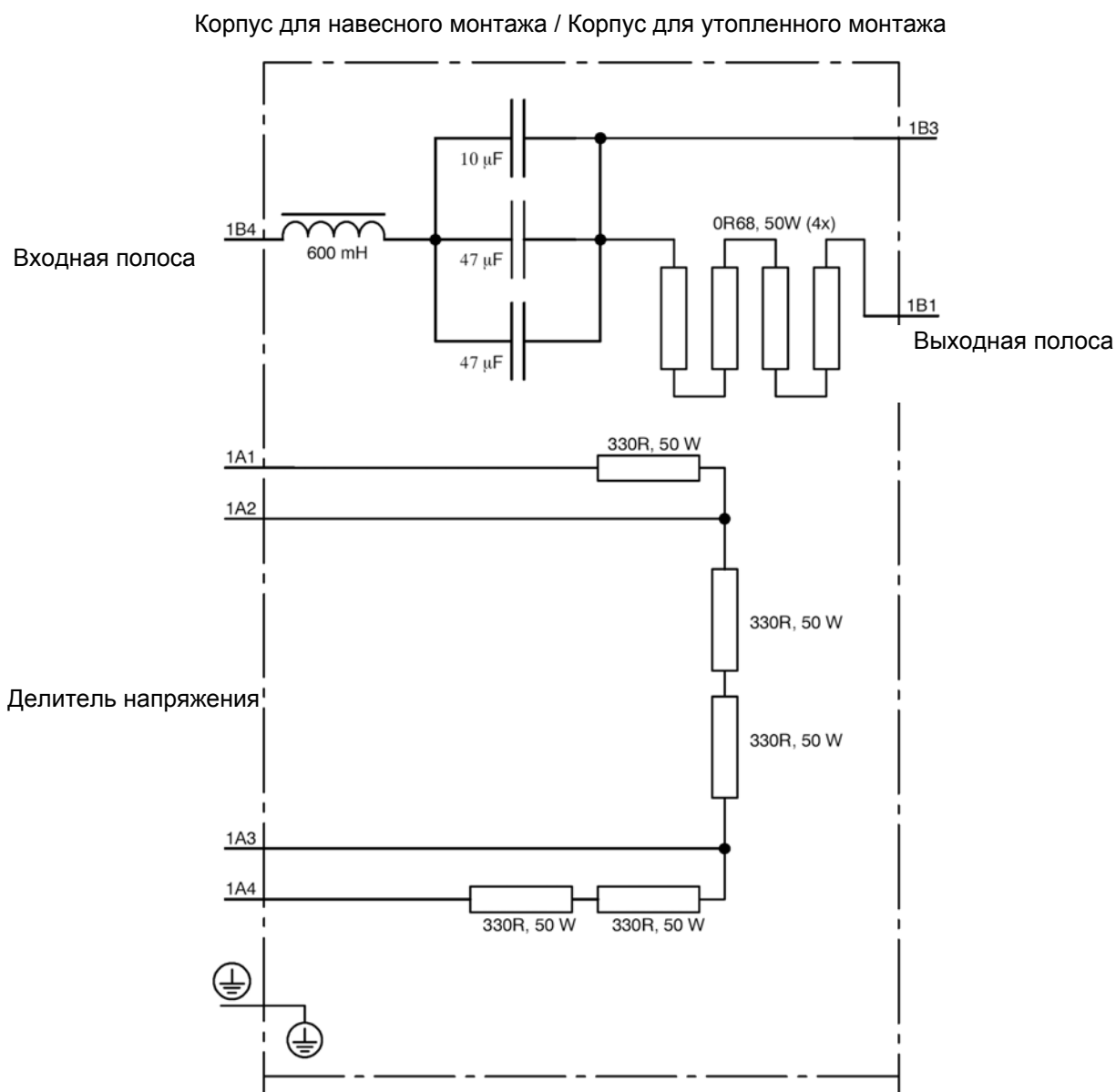
Рисунок 5 Общая схема 7ХТ3400-0*А00/DD
