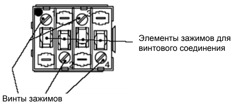
Рисунок 1 Подключение модуля напряжения
