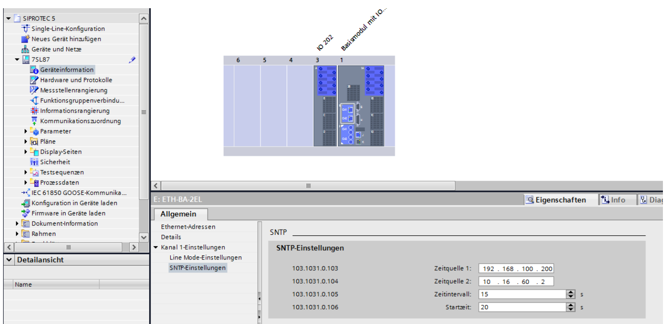
Bild 2: Einstellungen des Zeitserver bei SNTP in Verbindung mit Ethernet basierenden Protokollen
