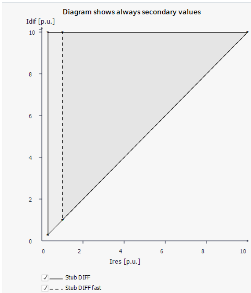
Abbildung 5: Eigenschaften Endfehler-Differentialschutz
