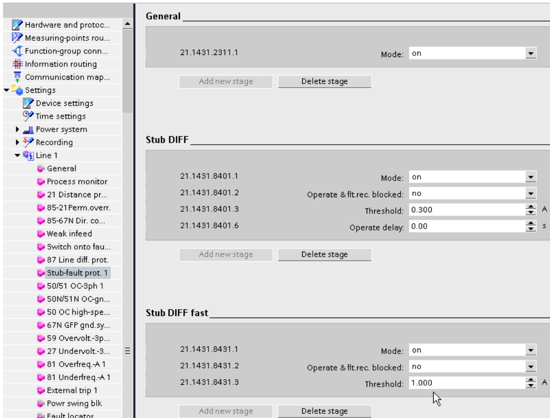
Abbildung 3: Einstellungen Endfehler-Differentialschutz
