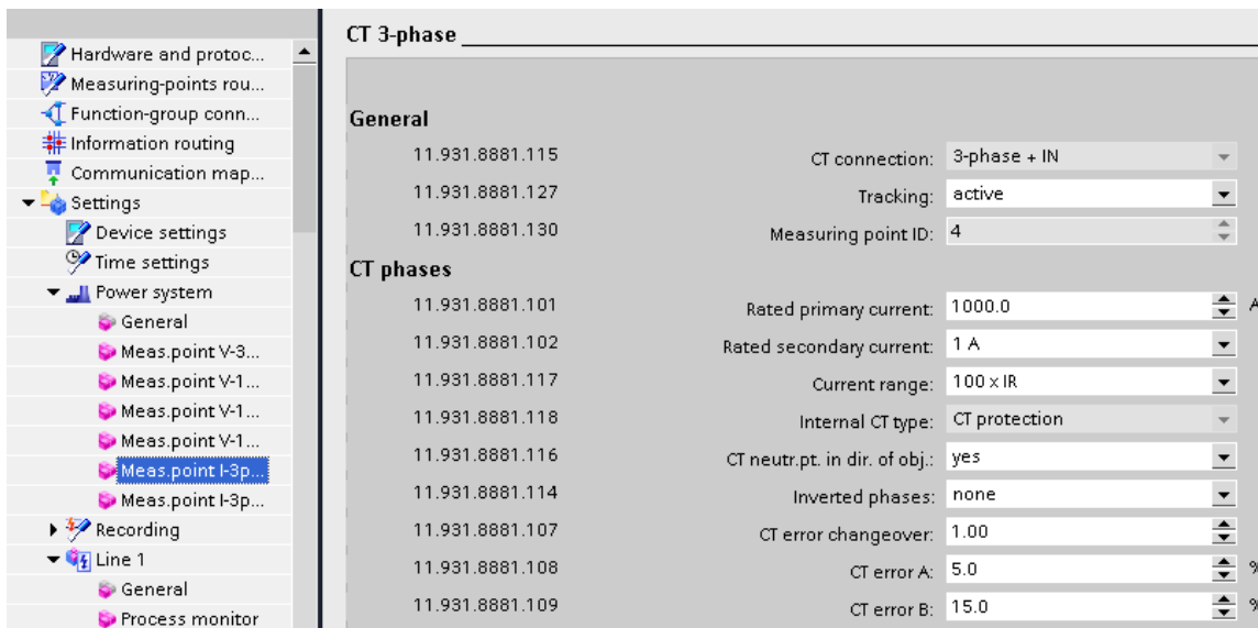
Abbildung 4: Einstellung CT-Fehler
