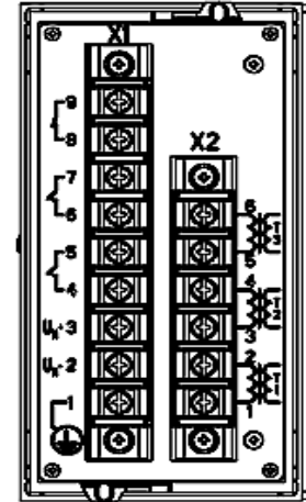
Bild 1-3 Geräterückseite Anschlüsse 7SJ46
