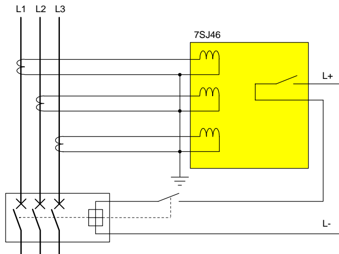
Bild 1-22 Anschluss 7SJ46 bei 3-Wandlerschaltung
