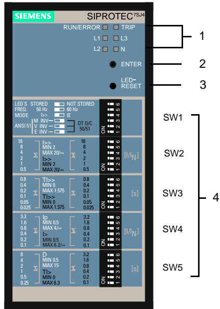
Bild 1-1 Gerätefront Bedien- und Anzeigeelemente des 7SJ46
