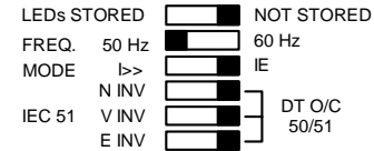
Bild 1-5 Grundeinstellungsblock, Beispiel IEC-Gerät
