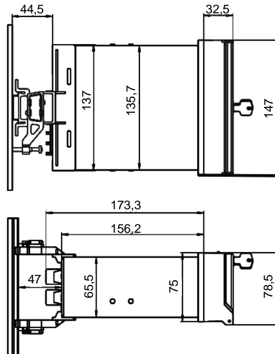
Bild 1-8 Hutschiennenmontage
