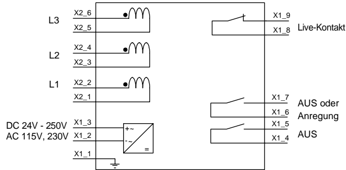
Bild 1-9 Anschlussplan 7SJ46
