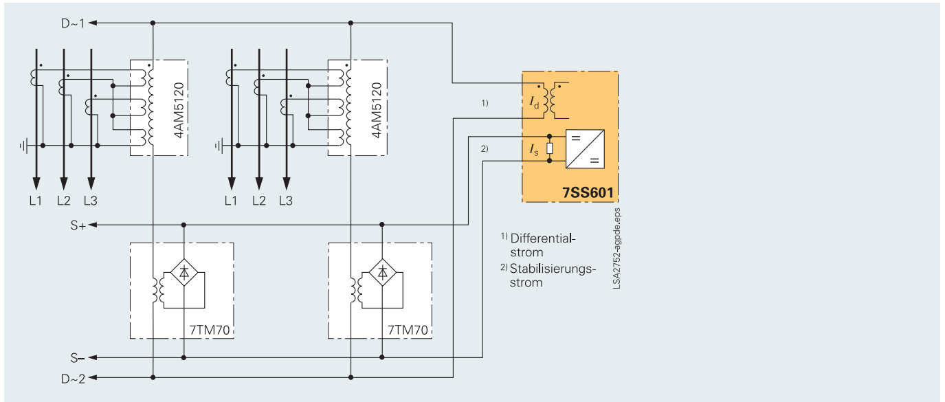
Abb. 9/6 Funktionsschema: Messwerterfassung
