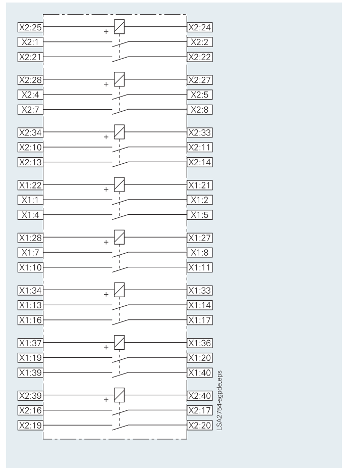
Abb. 9/16 Anschlussplan für 7TS720
