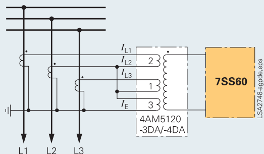
Abb. 9/8 Mischwandler-Variante (Stromkreis L1-L2-N)
