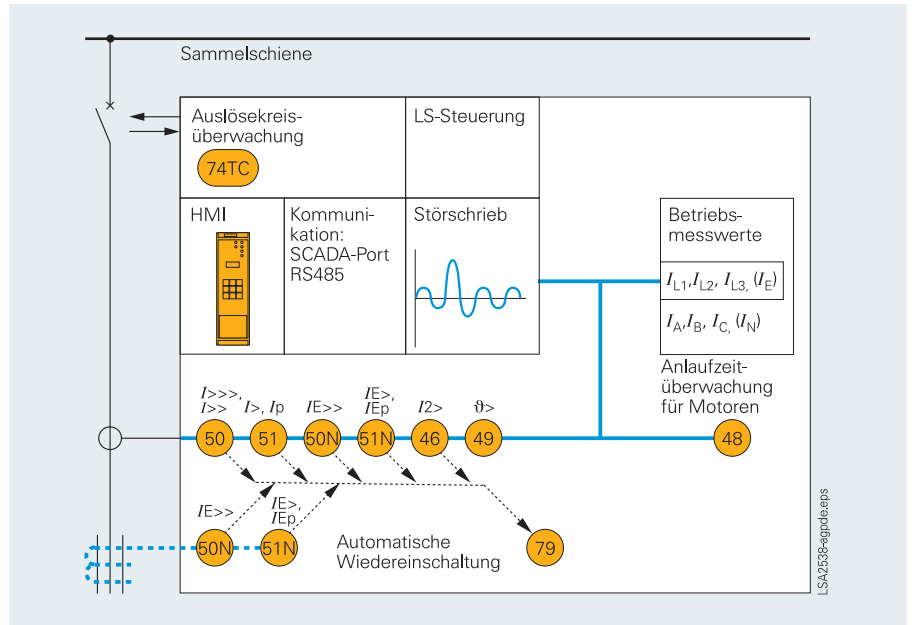
Abb. 5/20 Funktionsdiagramm
