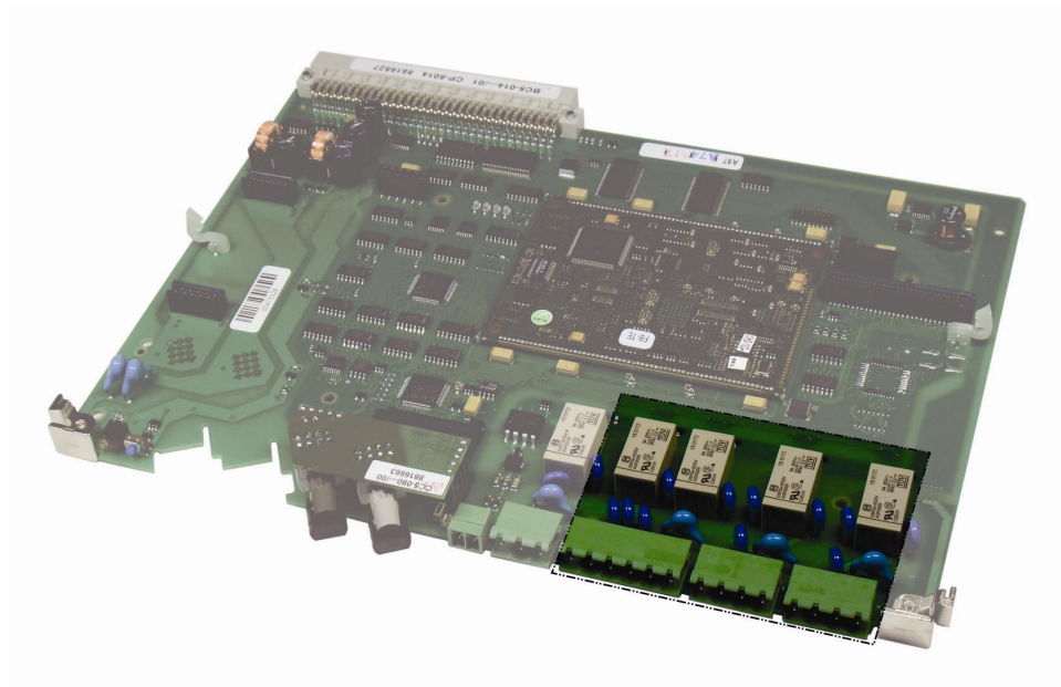
DO-5299 integriert in CP-5014
