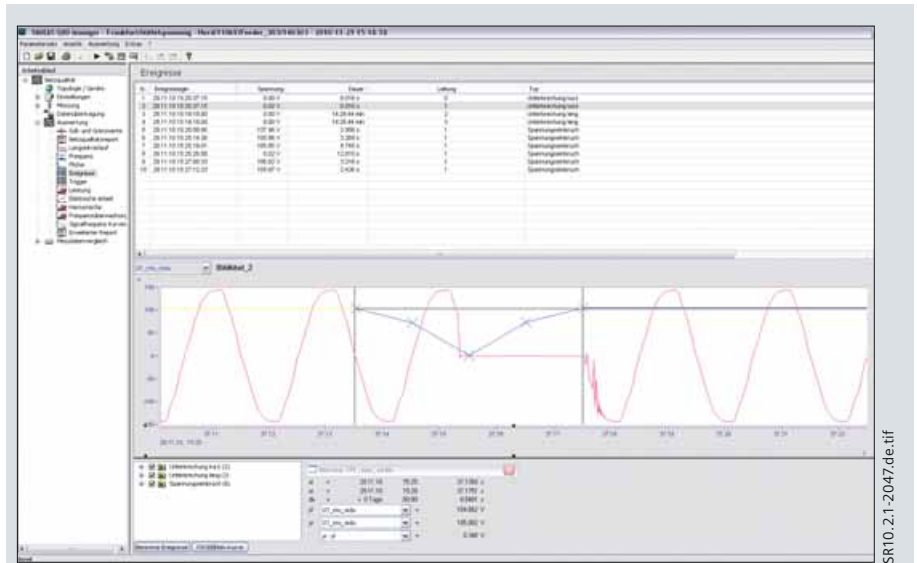
Bild 11 Spannungseinbruch
