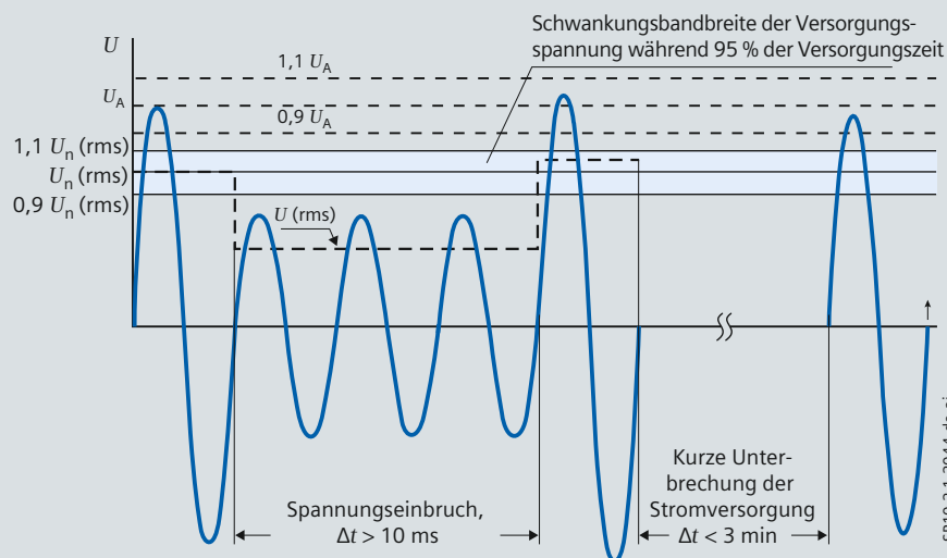
Bild 6 Darstellung eines Spannungseinbruchs und einer kurzen Unterbrechung der Stromversorgung mit Klassifizierung gemäß EN 50160; U_n – Nennspannung der Stromversorgung ( U_{eff} ), U_A – Amplitude der Versorgungsspannung, U_{eff} – Effektivwert der Versorgungsspannung
