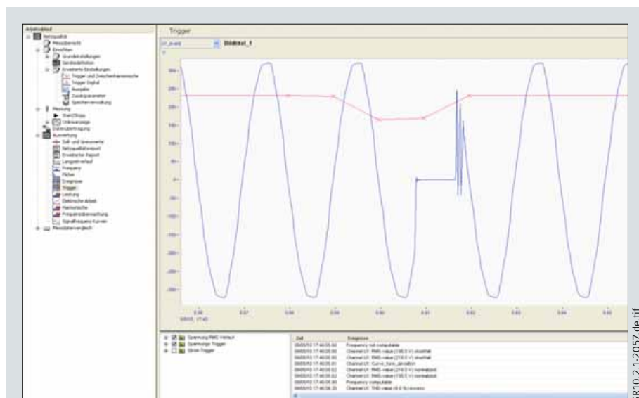
Bild 21 Trigger-Analyse
