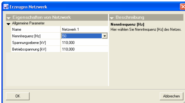
Bild 3-7 Power System Description, Netzwerk parametrieren
