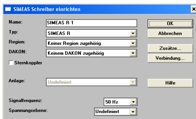
Bild 3-3 Dialog SIMEAS Schreiber einrichten
