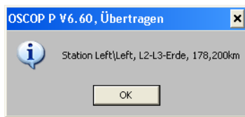
Bild 5-11 Ergebnismeldung der Fehlerortung
