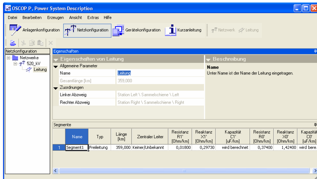
Bild 5-10 Netzkonfiguration mit parametrierter Leitung
