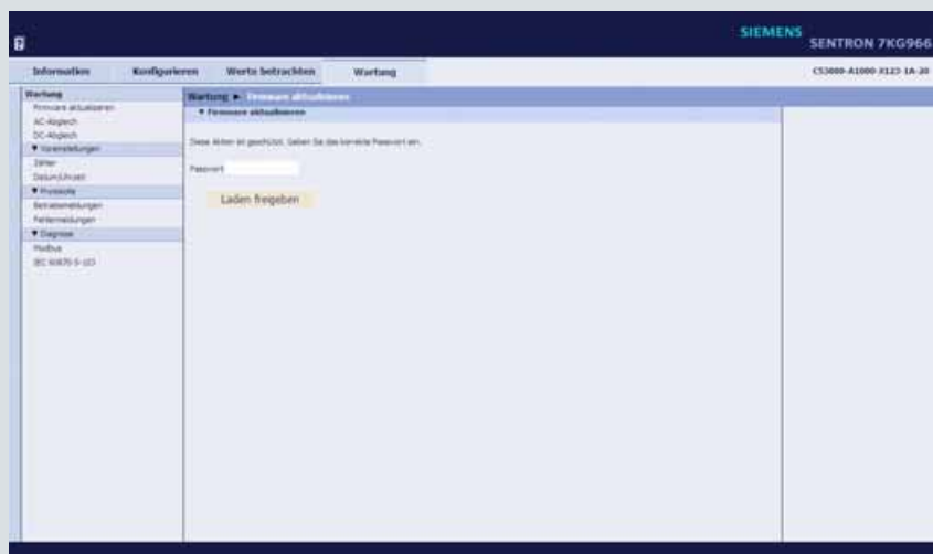
Fig. 11 Registerkarte Wartung
