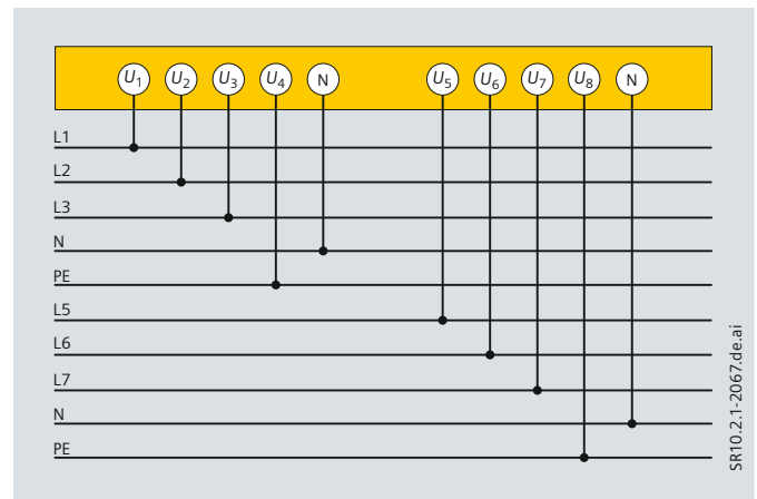
Bild 4/25 Konfiguration mit 8 Spannungsanschlüssen
