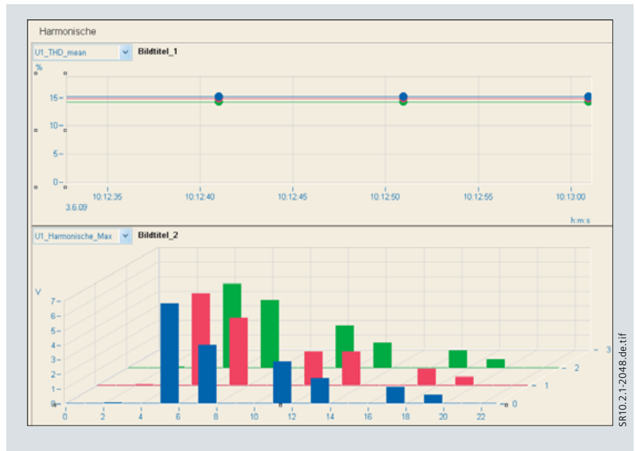
Bild 4/11 Übersicht Oberschwingungen
