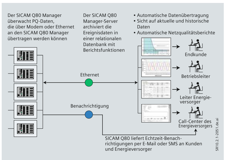
Bild 4/14 SICAM Q80 – Systemübersicht
