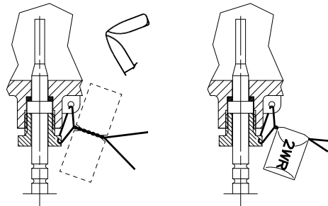
Abb. 7: Beispiel Vorlauffühler
