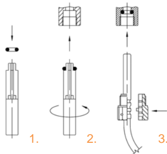
Abb. 3: Montage Adapterset
